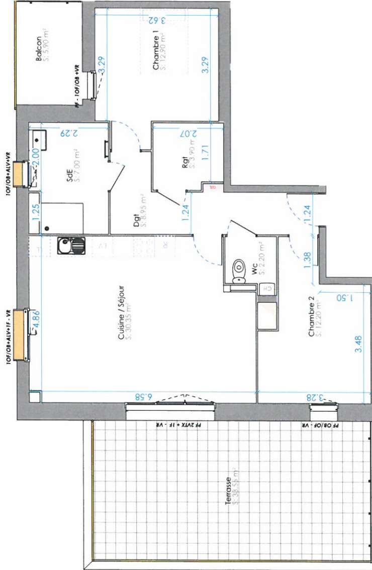
PLAN R+2
